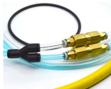
Tubi di raccordo al mono dotata di valvola a due vie con non ritorno
